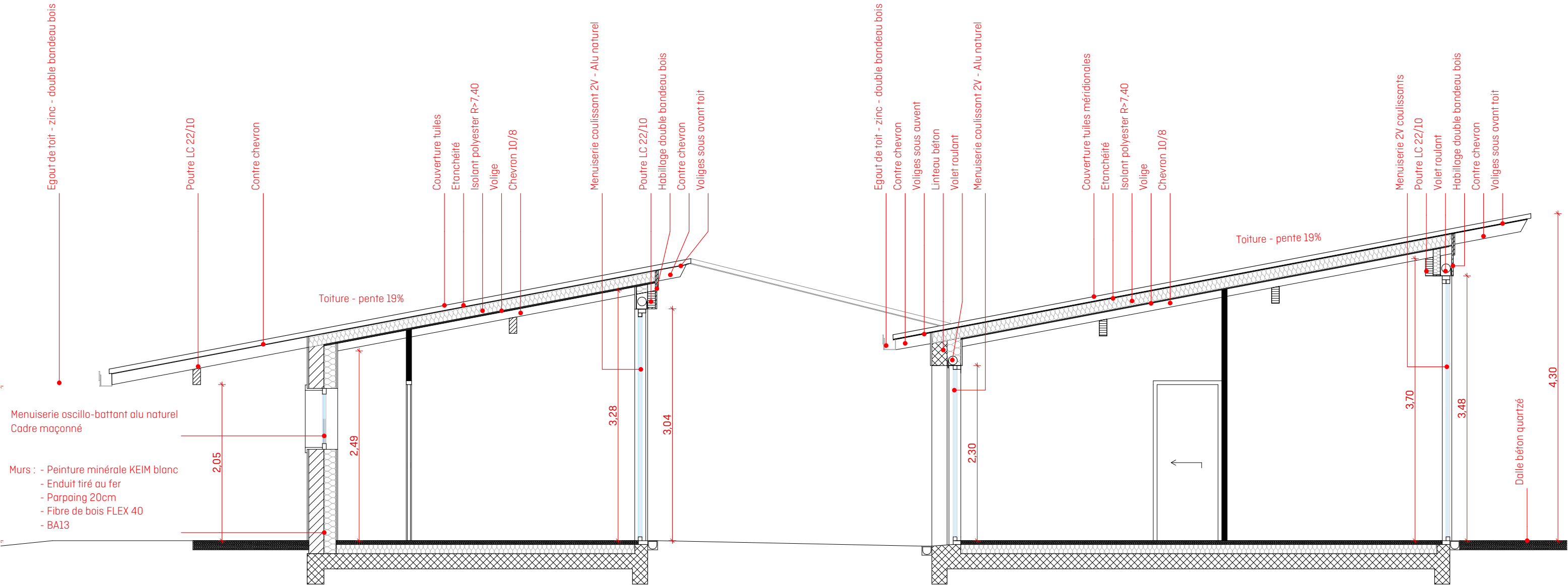
Coupe BB - éch. 1/50
