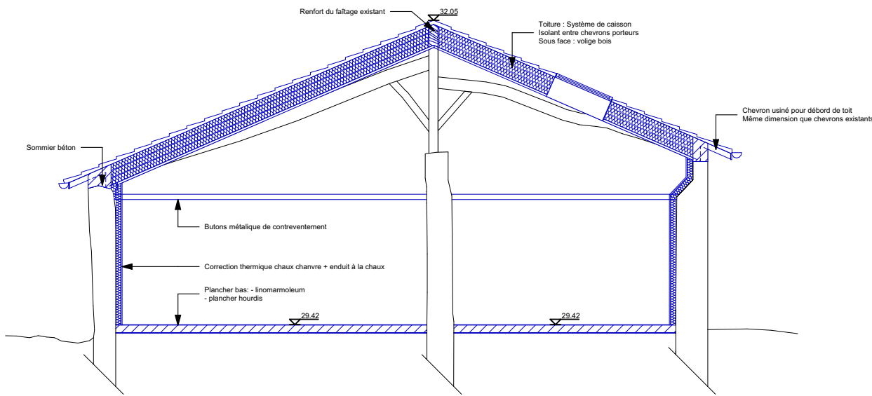
COUPE TRANSVERSALE SUR LA MAM
