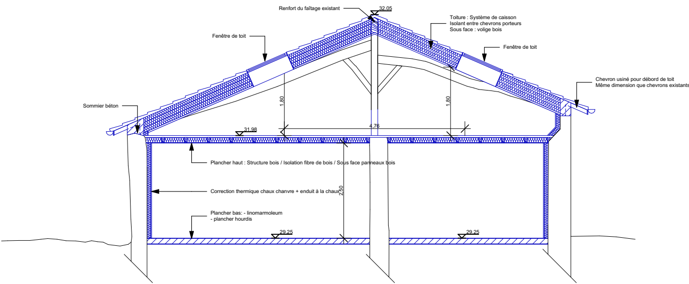
COUPE TRANSVERSALE SUR LOGEMENTS
