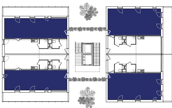
AZAR . ÉTAGE COURANT . UNITÉS ANNEXES
