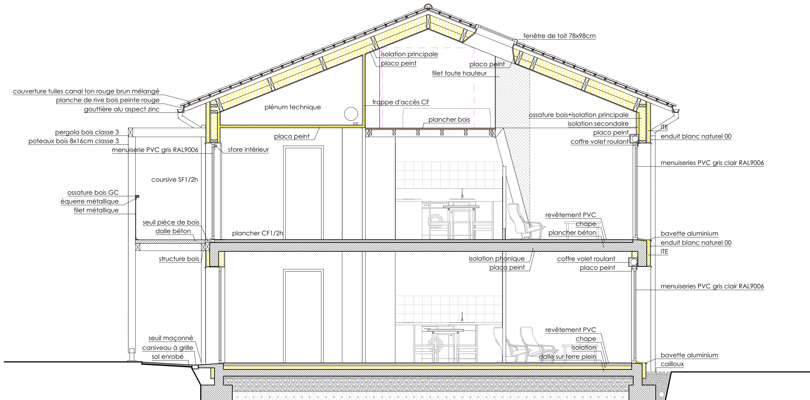
Coupe AA
