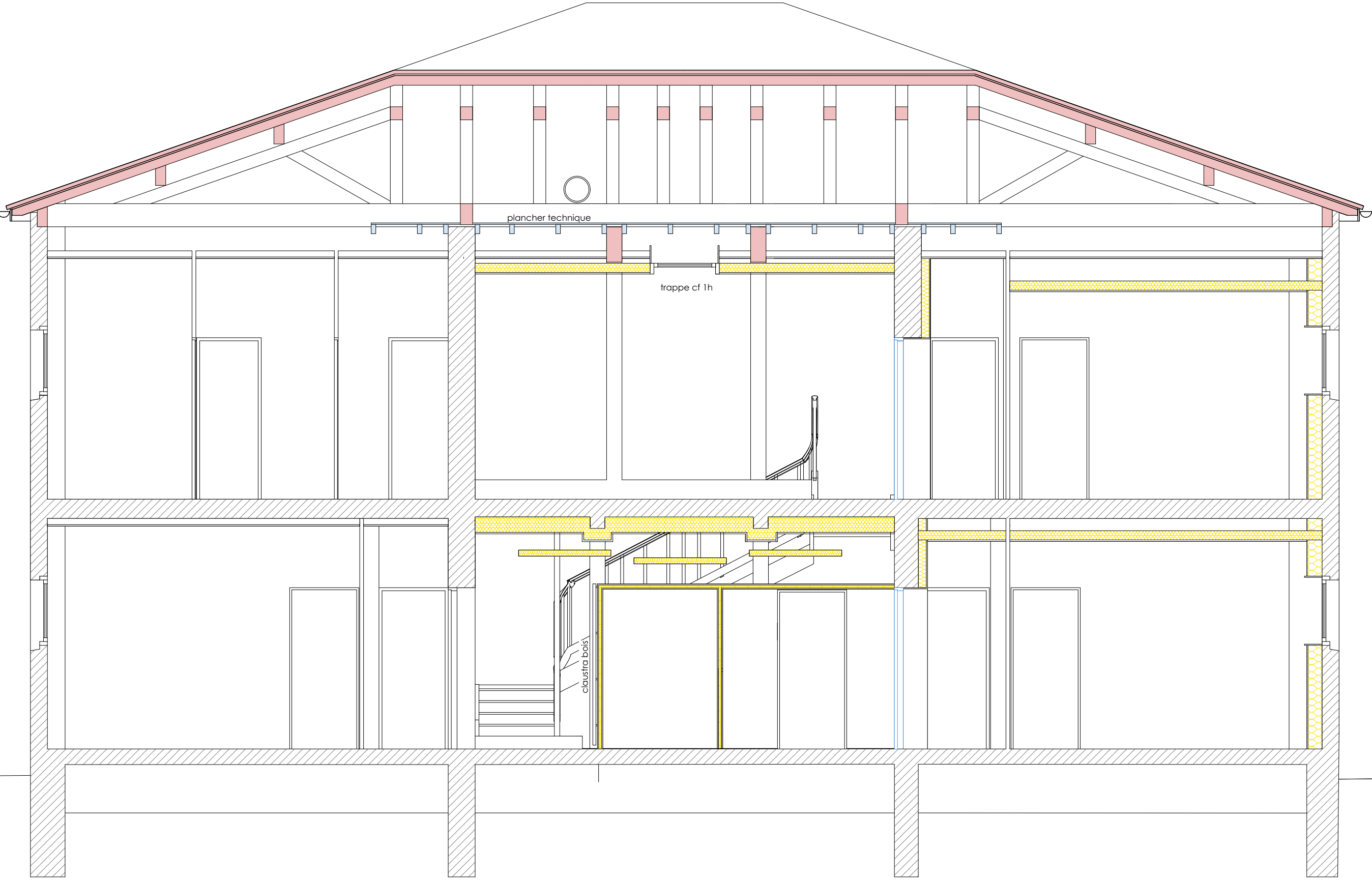
Coupe Projet
