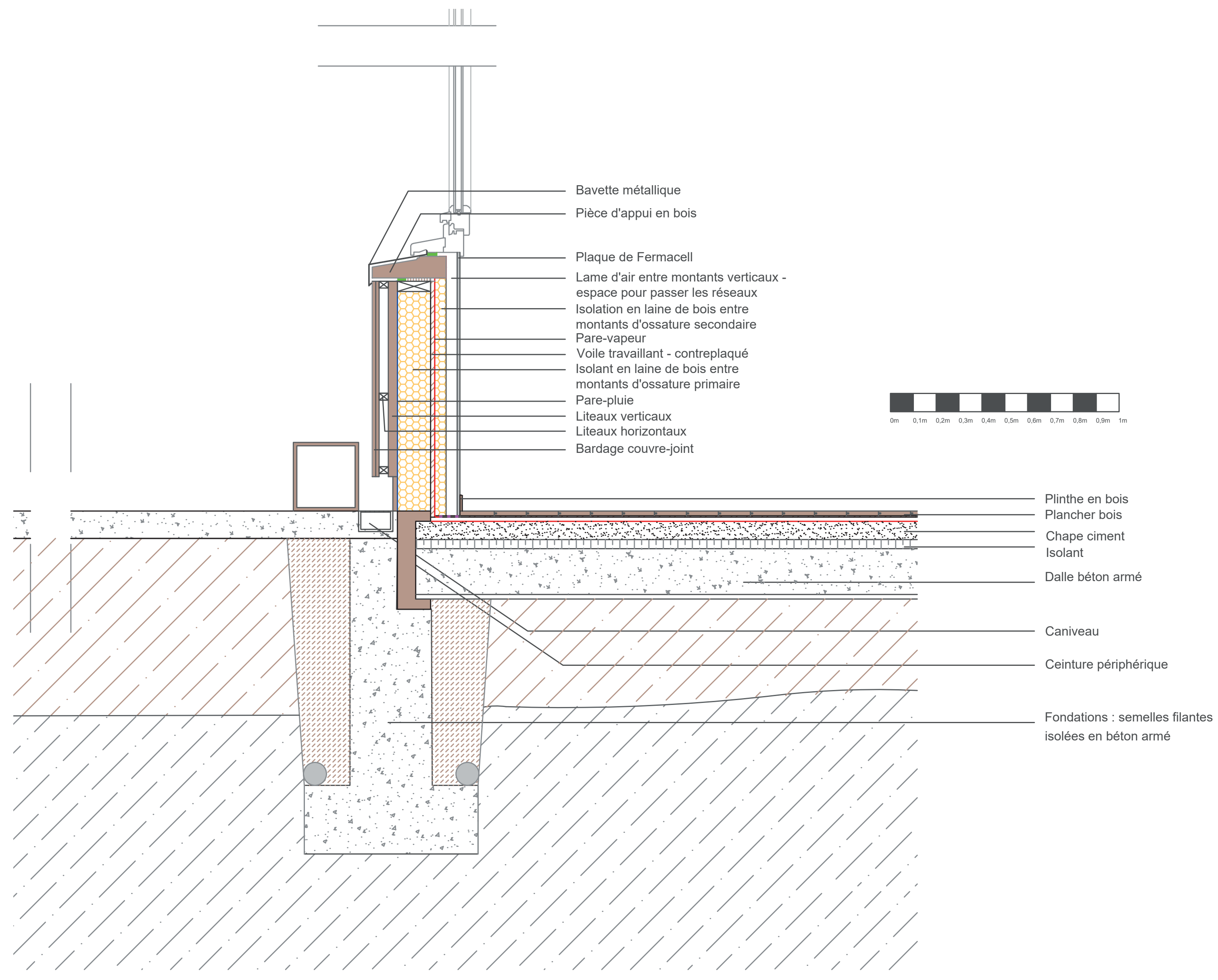
Coupe de détail de la paroi ossature bois de l'extension neuve
